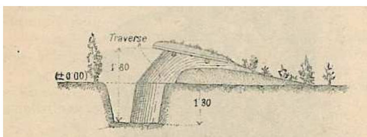
Obr. 1/3: Řez nakrytým zákopem. Nejedná se o totožný typ jako na obr. 1/2. Zákop na výkrese je opatřen traverzami a nejsou zde zakresleny svislé podpěry.
